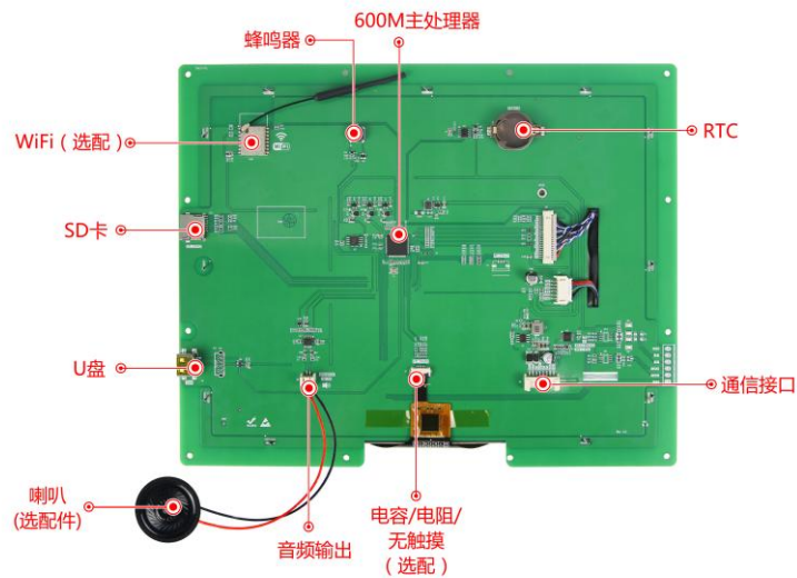
图 1-4 硬件配置图
