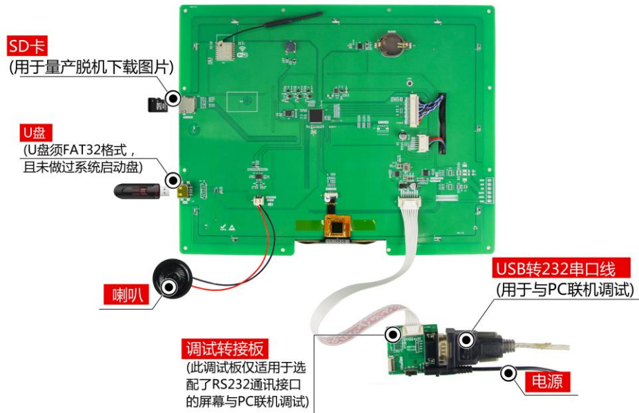
图 1-5 调试工具图
