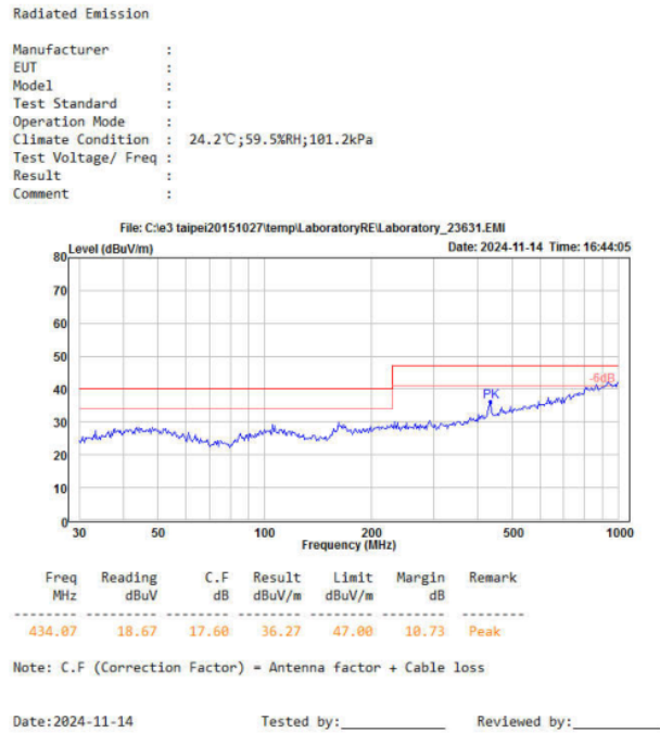
图 4-5 RE 测试水平方向
